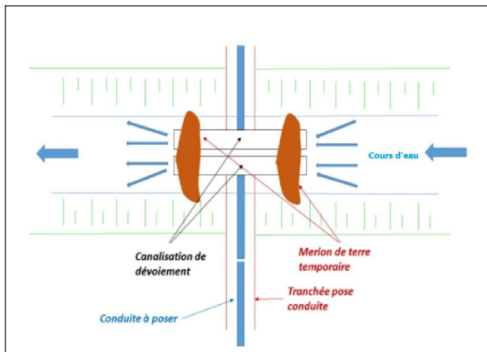
Schéma type du dispositif mis en place pour une traversée de cours d'eau
