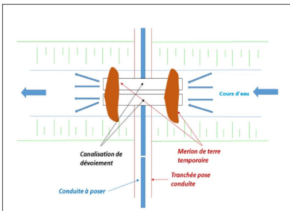
Figure 1 : schéma type du dispositif mis en place pour une traversée de cours d'eau
