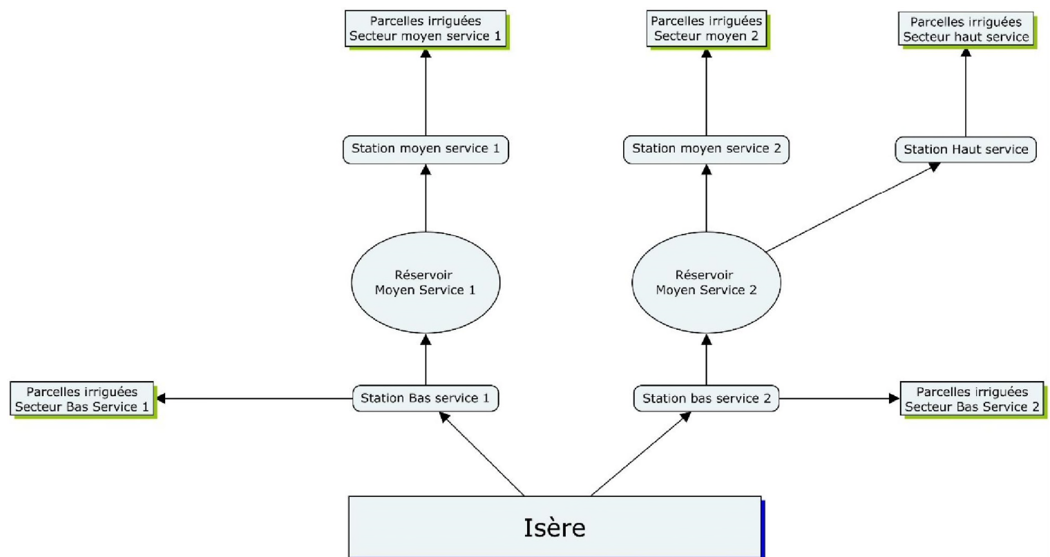
Figure 3 Schéma synoptique de la distribution sous pression (CA-EAU)
